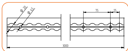
Uniwersalne rozmieszczenie otworów.
