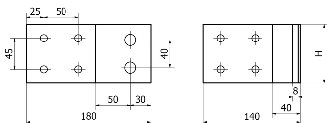
Naroża aluminiowe uniwersalne z otworami przesuniętymi pod profil słupa Jekl (60x30).
