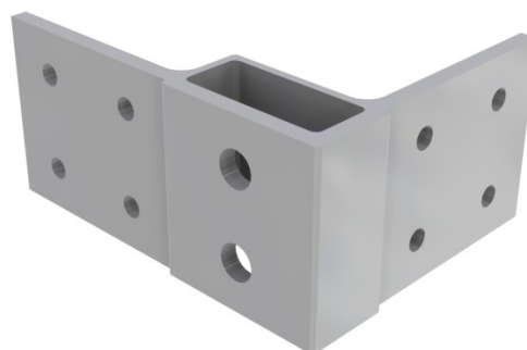
Naroża aluminiowe uniwersalne z otworami centralnymi pod profil słupa 80x35.
