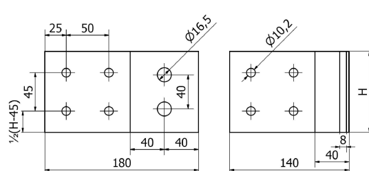
Naroża aluminiowe uniwersalne z otworami centralnymi pod profil słupa 80x35.
